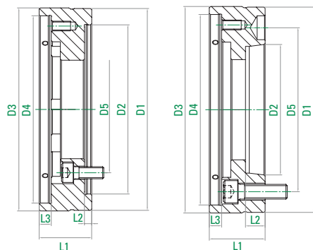
Zwischenflansche
