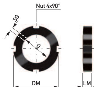
Abdrückmutter mit Verdrehsicherung Nutmutter ähnlich DIN 1804 mit Sicherungsgewinde und Gewindestift
