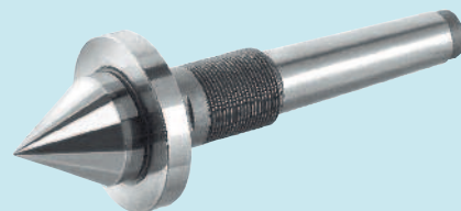
Zentrierspitze mit Messbund
